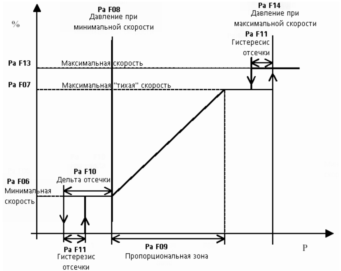
Диаграмма управления вентиляторами
