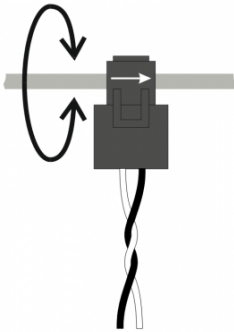
Подключение выводов токовых трансформаторов
