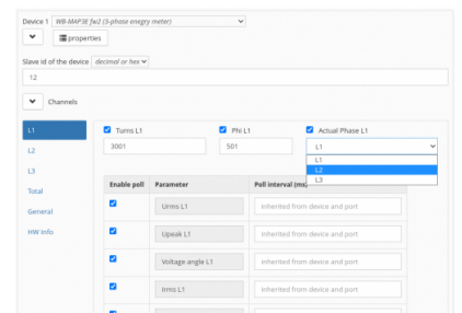
Настройка токовых трансформаторов и маппинга фаз в параметрах счётчика WB-MAP3E в веб-интерфейсе контроллера Wiren Board
