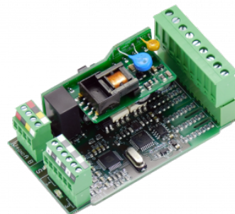
Плата WB-MAP3E
